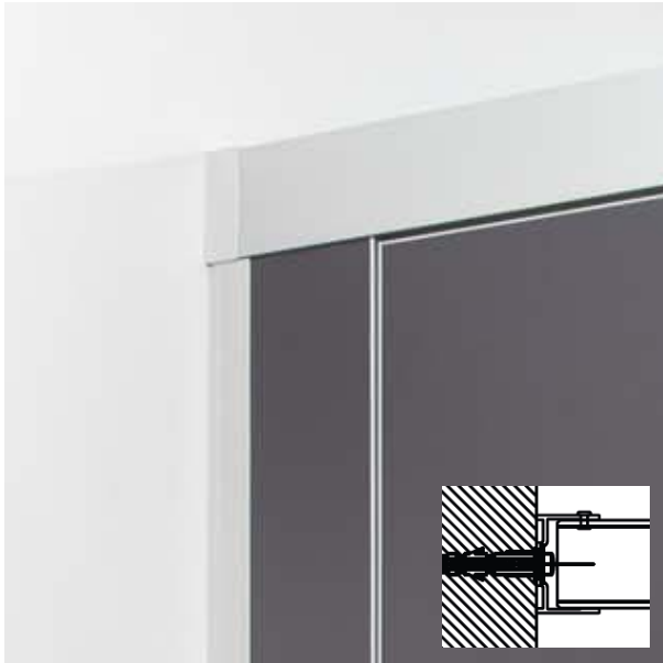
Maueranschlüsse durch U-Profile zum Ausgleich von Bauleranzen
